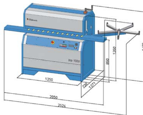
Рис. 2. Габариты станка, модель TOP 1000
