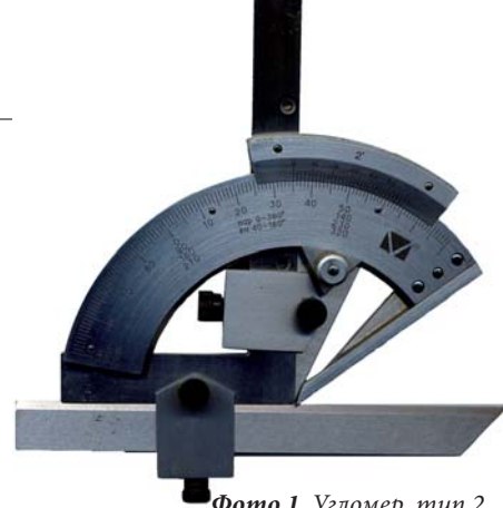
Фото 1. Угломер, тип 2
