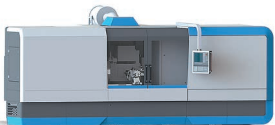
☞ Универсальный круглошлифовальный станок с ЧПУ модели ОШ-660.3.Ф3
